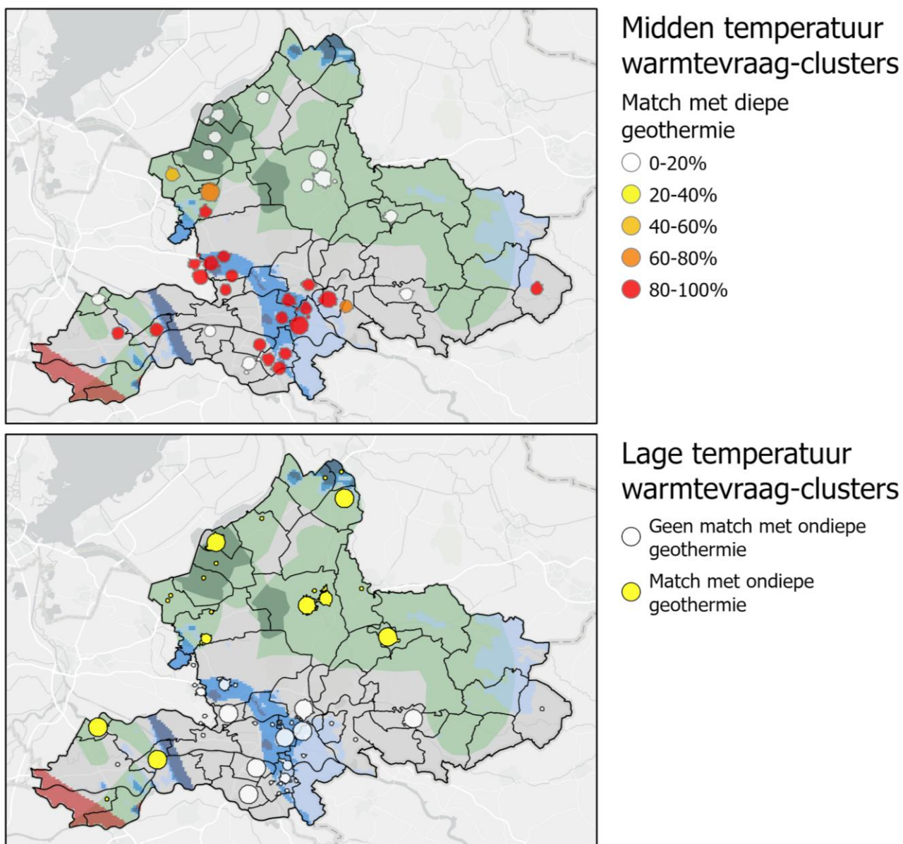
Afbeelding 0.3 Percentage van de midden (boven), en lage (onder) temperatuur warmtevraag dat met diepe of ondiepe geothermie kan worden geleverd in enkele zones (gekleurde cirkels) waar de warmtevraag relatief hoog is. 1,2,3
