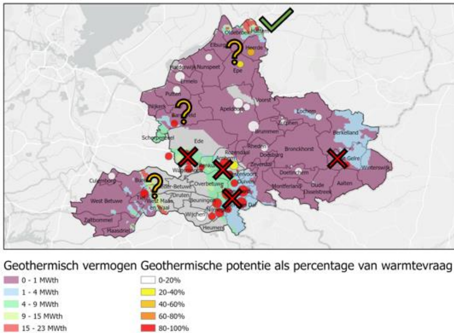
Afbeelding 5.6 Invulling van de warmtevraag (in %) in verschillende gebieden in Gelderland waar deze relatief hoog is (cirkels) door middel van diepe geothermie (Rotliegend Formatie, Mid Case). In de grijze gebieden komt het Rotliegend niet voor.
