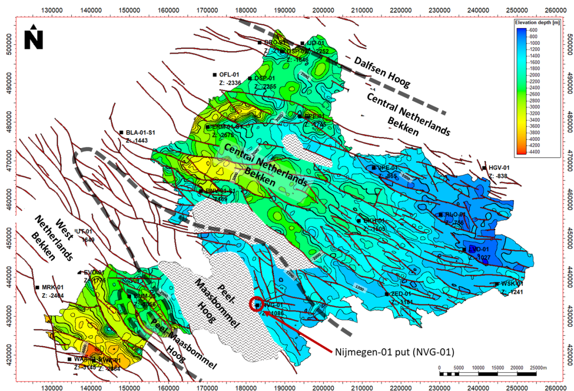
Abbeelding 5.3 De diepte kaart van de top Rotliedend, contour interval 200 m. In het noordwesten van Gelderland ligt het Rotliedend dieper dan in het zuidoosten. In de gearceerde vlekken is het Rotliedend afwezig (geërodeerd)
