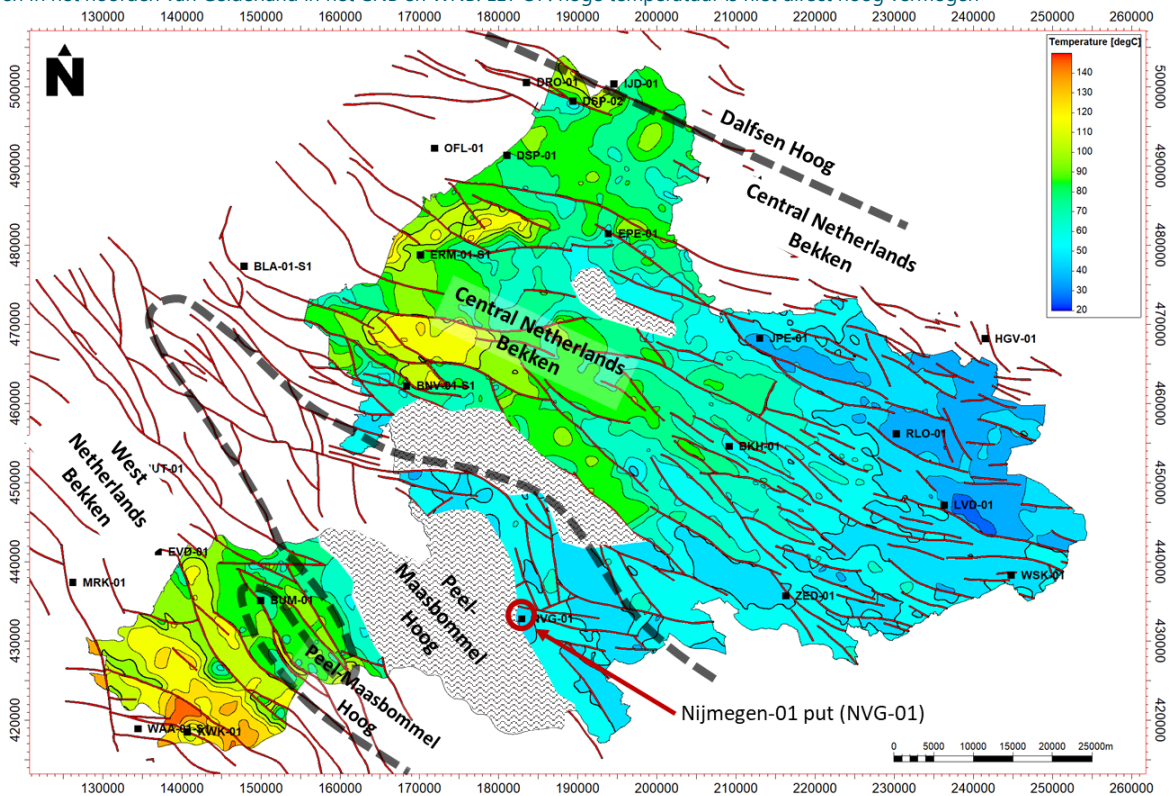
Abbeelding 5.4 De temperatuurkaart van het Rotliedend toont hoge temperaturen van 100 °C en meer in het westen (de Betuwe) en in het noorden van Gelderland in het CNB en WNB. LET OP: hoge temperatuur is niet direct hoog vermogen
